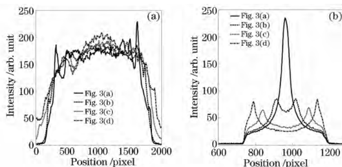
图 4 圆形光纤在不同入射偏移量条件下的(a)远场和(b)近场截面光强分布
