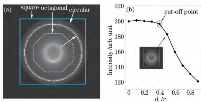
图 7 (a) 圆形结合多边形光纤传输系统中的芯径差异;(b) 圆形结合八边形光纤传输系统中入射偏移引起的能量损失
